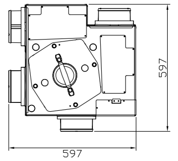
澄家VS80 熱交換率:80%
